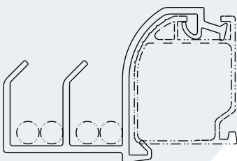
BP3-Kabelführung Artikel-Nummer: 105012004
