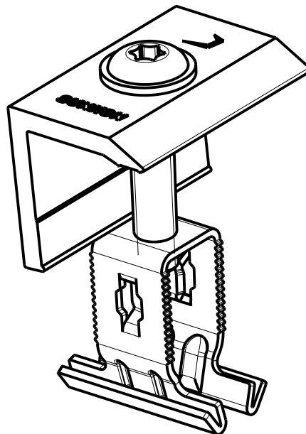
Endklemme Alu-ELP schwarz Artikel-Nummer: 105004003
