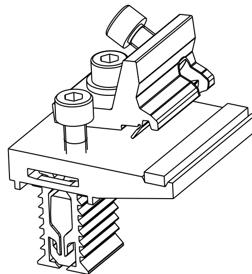
Höhenverstelleinheit parallel Artikel-Nummer: 105006002
